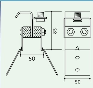
スーパードリッパⅢ S-60 葺替用 NKR300
