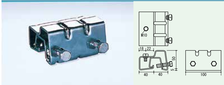
スーパーサドルW
