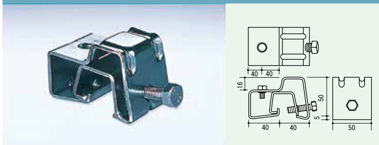
スーパーサドルS
