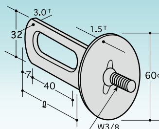
ツバ付足
