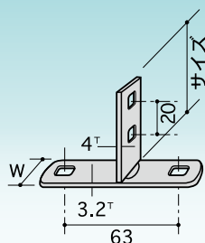
T字足
