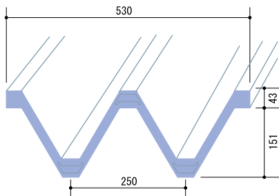
150 すきま面戸 二連 H-43
