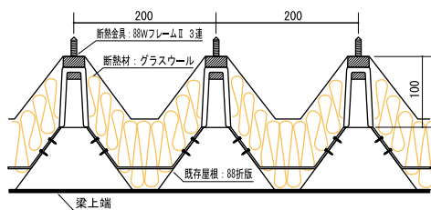
88スーパーWフレーム II H-100
