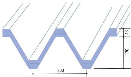
S-60 すきま面戸 H-43
