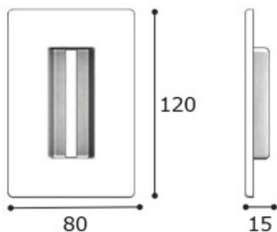
製品寸法
