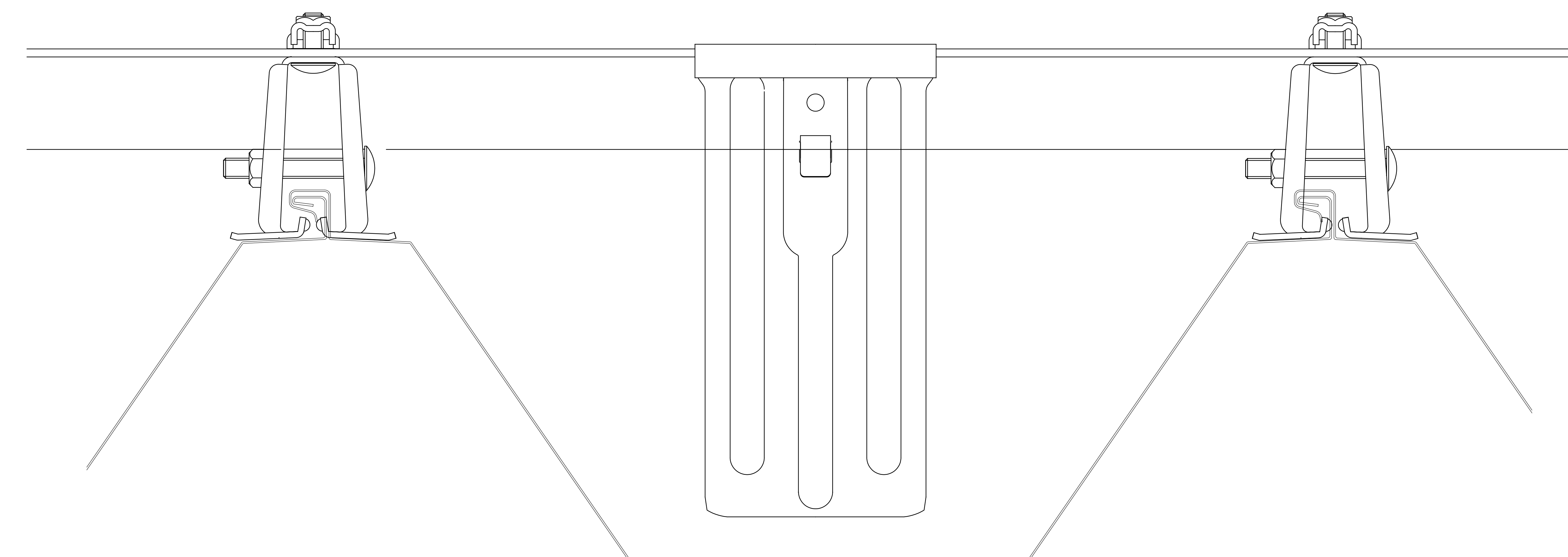
KBハゼ500型施工 雪止アンクルL4x50x50 + 神通F - 1 + ワンタッチバレーガードOT-5
