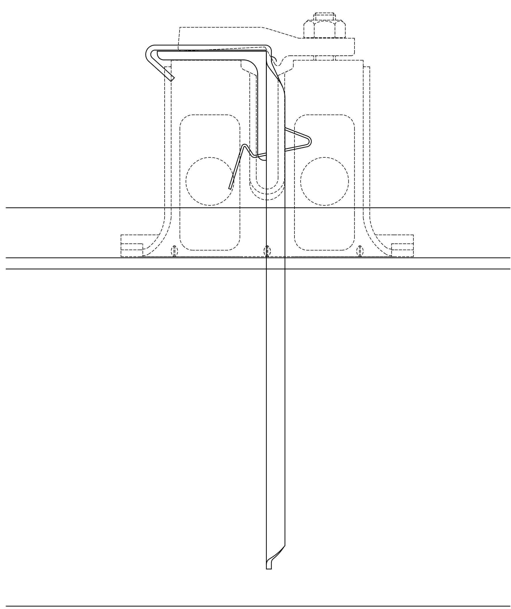
KBハゼ500型施工 雪止アンクルL4x50x50 + 神通F - 1 + ワンタッチバレーガードOT-5
